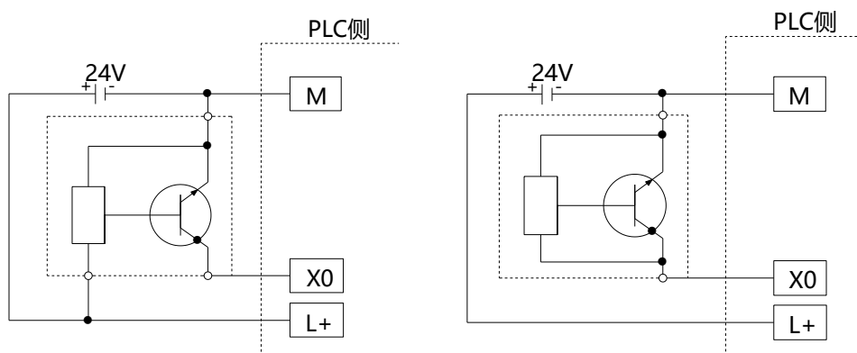
三线制 (NPN 型) 接近开关接线图示例
