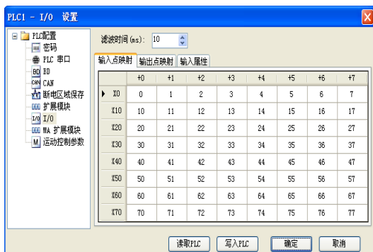
信捷PLC编辑软件I/O设置界面
