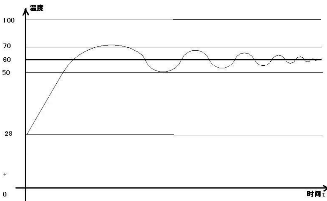
图 4 PID 自整定允许超调波形图
